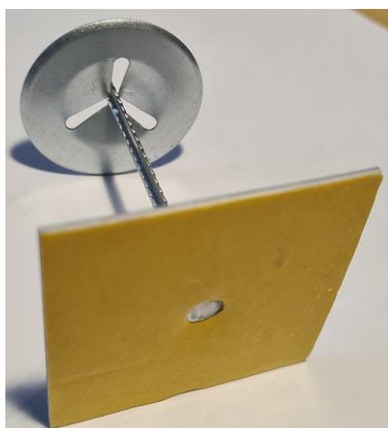
Avdragbart skyddspapper. Låsbricka Ø38 mm.
