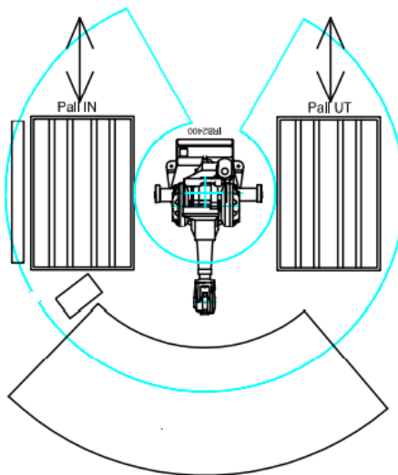
Exempel på layout av komplett cell.
