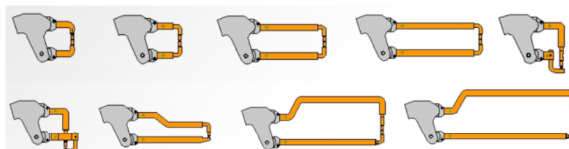
Exempel på armar till X- tänger.
