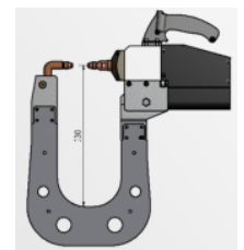
Exempel på arm till C-tänger (finns med olika djup).
